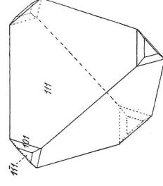
Fig. 50. Helvin, \{110\} , \{111\} , \{1\bar{1}\bar{1}\} , Hørtokollen.
