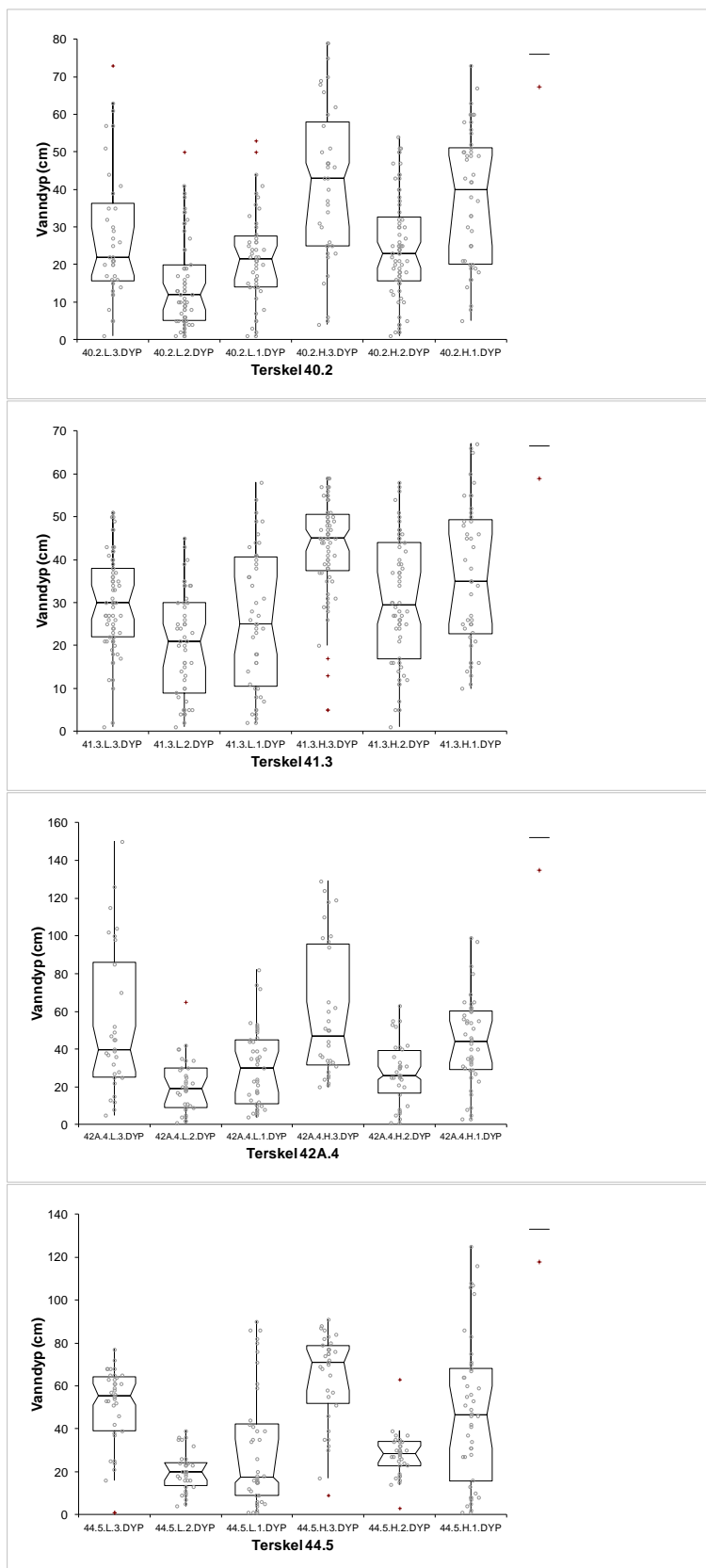
Figur 25. Box-plot diagram for innmålte vanddyb på alle tre transekter og per terskel ved hhv lav (ca. 2,5 \text{ m}^3 \text{ s}^{-1} ; tre transekter til venstre) og høy (ca. 12,5 \text{ m}^3 \text{ s}^{-1} ; tre transekter til høyre) vannføring. Midtlinjen viser medianverdien, øvre linje viser 75 % percentilen og nedre 25 % percentilen og kryssene viser uteliggende verdier.
