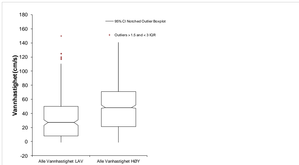
Figur 29. Box-plot diagram for innmålte vannhastigheter på 12 transekter ved hhv lav (ca. 2,5 \text{ m}^3 \text{ s}^{-1} ) og høy (ca. 12,5 \text{ m}^3 \text{ s}^{-1} ) vannføring. Midtlinjen viser medianverdien, øvre linje viser 75 % percentilen og nedre 25 % percentilen og kryssene viser uteliggende verdier.
